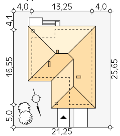
Gabaryty działki:
