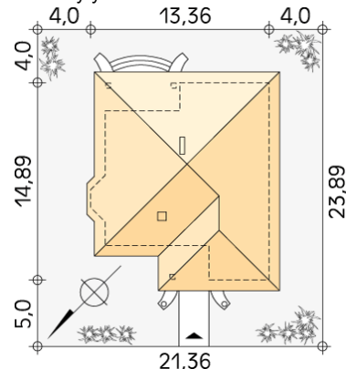
Gabaryty działki:
